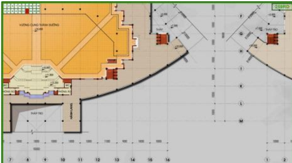
G LẦU 2 (COTE +10.000)
